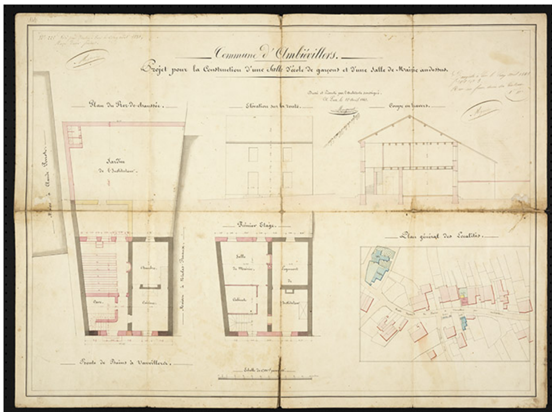
Projet pour la construction d'une salle d'école des garçons et d'une salle de mairie.
