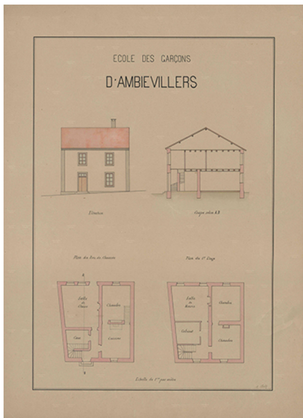
Plan de l'école des garçons : élévation, coupe, plan du rez-de-chaussée, plan du 1er étage.
