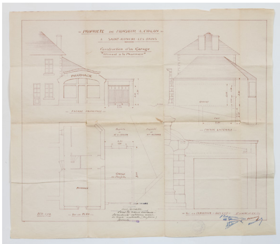
Plan et élévations du garage attenant à la pharmacie.
