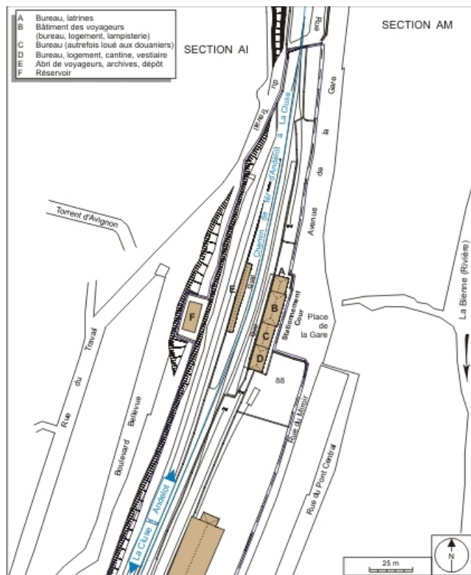
Plan-masse de la partie nord (gare des voyageurs).
