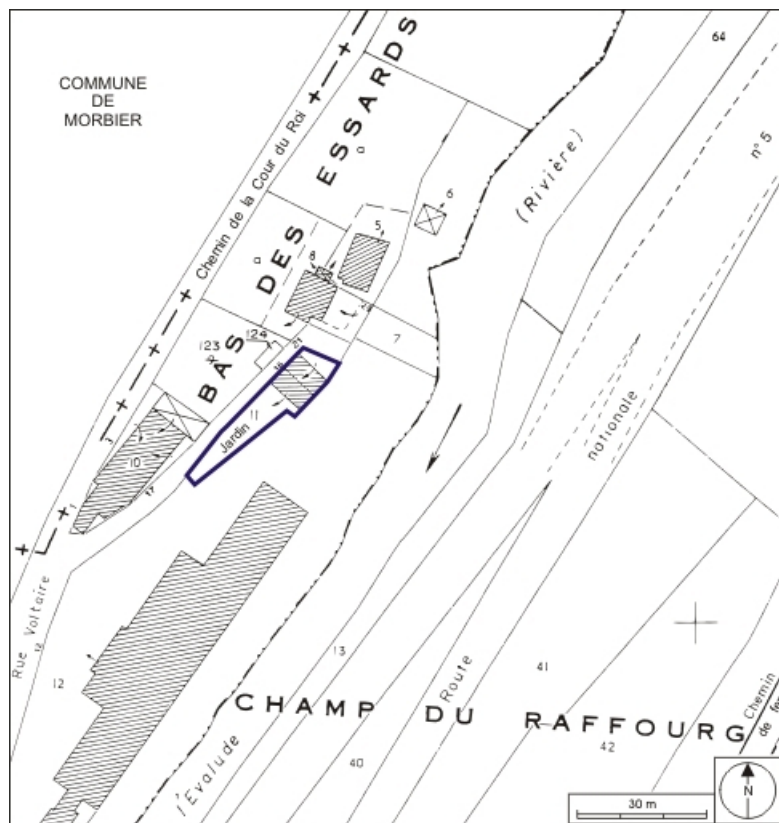
Plan-masse et de situation. Extrait du plan cadastral, 1980, section AC, échelle 1:1000. 39, Morez, 16 rue Voltaire
