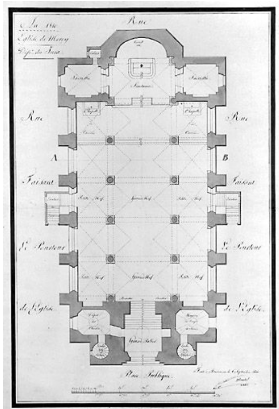
An 1810. Église de Morey [plan].
