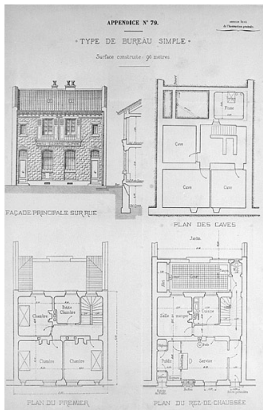
" Type de bureau simple " [projet type]. Façade principale sur rue, plan des caves, plan du rez-de-chaussée, plan du premier. 39, Molinges
