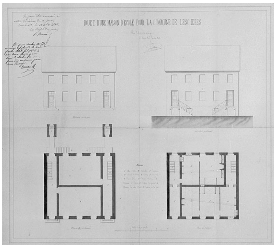
Projet d'une maison d'école pour la commune de Leschères [plans et élévations].
