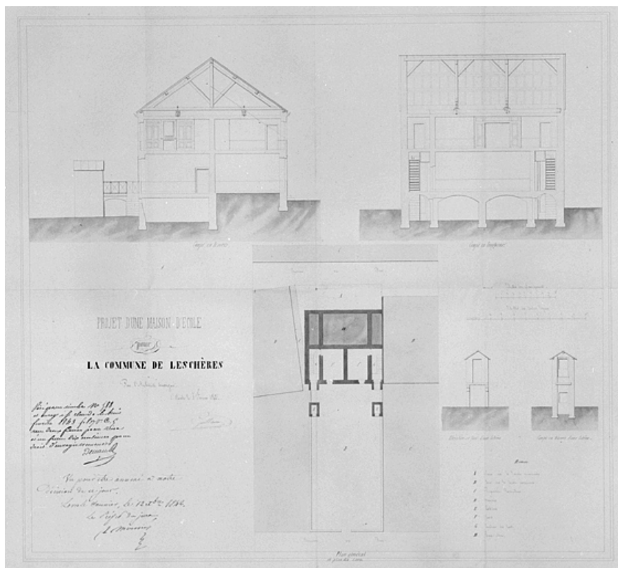
Projet d'une maison d'école pour la commune de Leschères [plan-masse et coupes]. 39, Leschères Ecole
