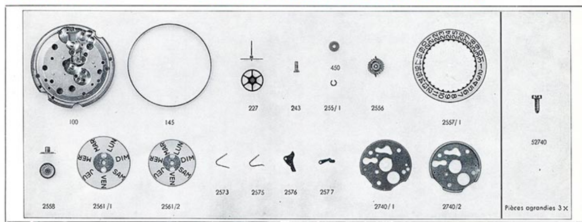
Calibre 11 1/2''' - 140-2 - Jour-date - (fournitures particulières), 1973.
