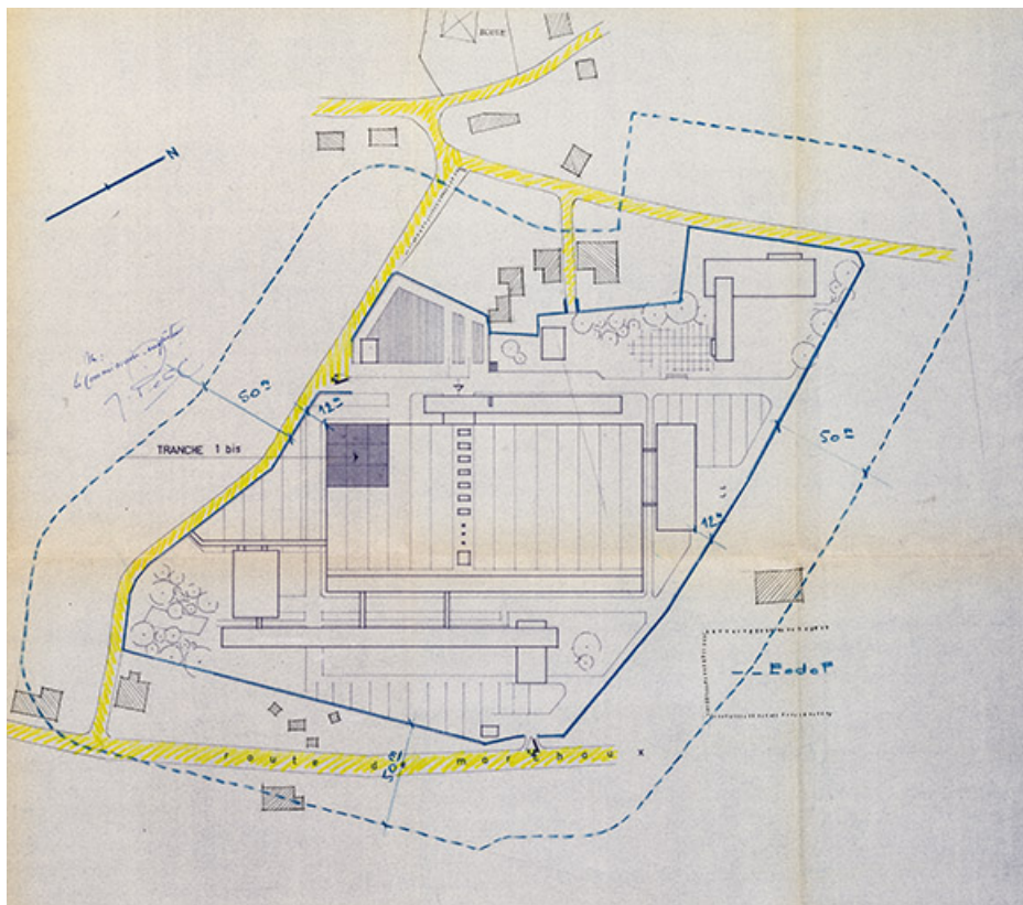
Usine de Palente. Plan-masse, 1957.
