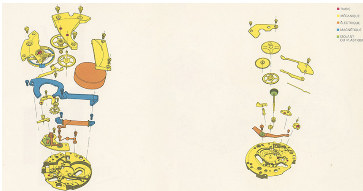
Eclaté d'un mouvement de montre Lip, 1969.
