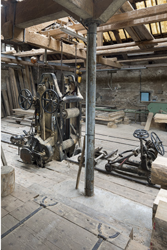
Atelier de fabrication : châssis de scie Socolest, vu de trois quarts gauche.
