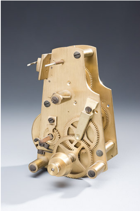
Mouvement de pendule Japy
