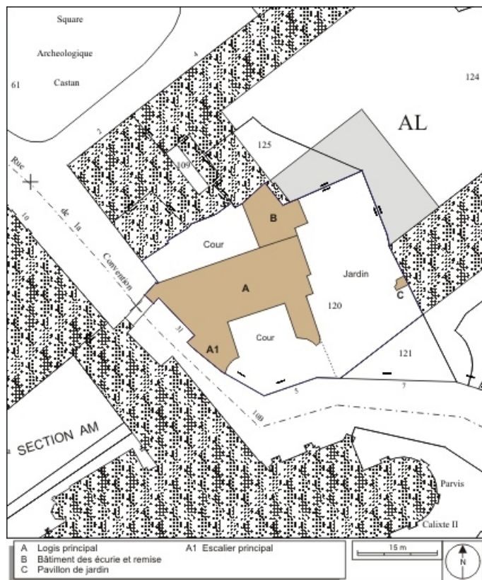
Plan masse et de situation. Extrait du plan cadastral, 1974, section AL. 25, Besançon, 3, 5 rue de la Convention, lieudit : îlot Boitouset
