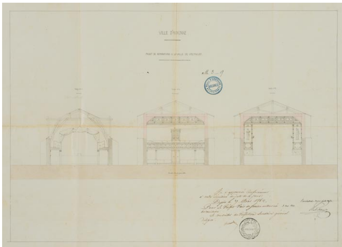
Ville d'Auxonne. Projets de réparations à la salle de spectacle. [Coupe transversale]. 3 mai 1842. 21, Auxonne boulevard Pasteur
