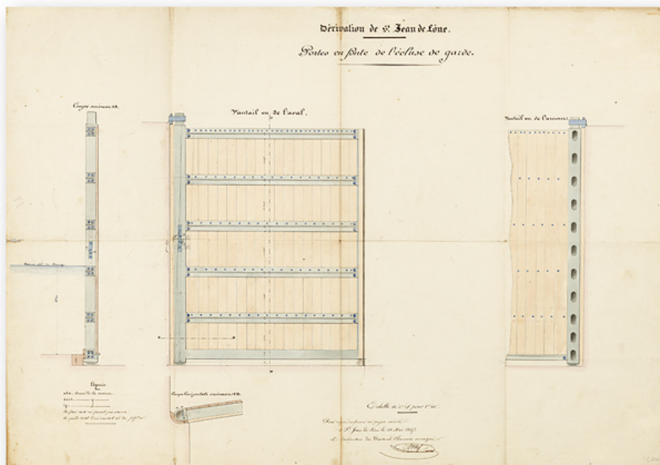
Portes en fonte de l'écluse de garde. Dessin daté du 28 mai 1847. 21, Saint-Usage, lieudit : PK 212
