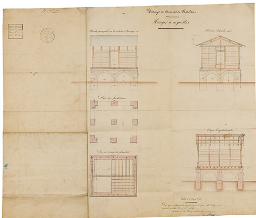
Barrages de Seurre et du Châtelet. Hangar à aiguilles. [Plan, coupe et élévation]. 17 octobre 1847.
