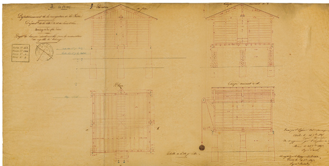
Projet de hangar insubmersible pour la conservation des aiguilles de barrage. [Plan, coupe et élévation]. 26 septembre 1847. 21, Pagny-la-Ville, lieudit : PK 200
