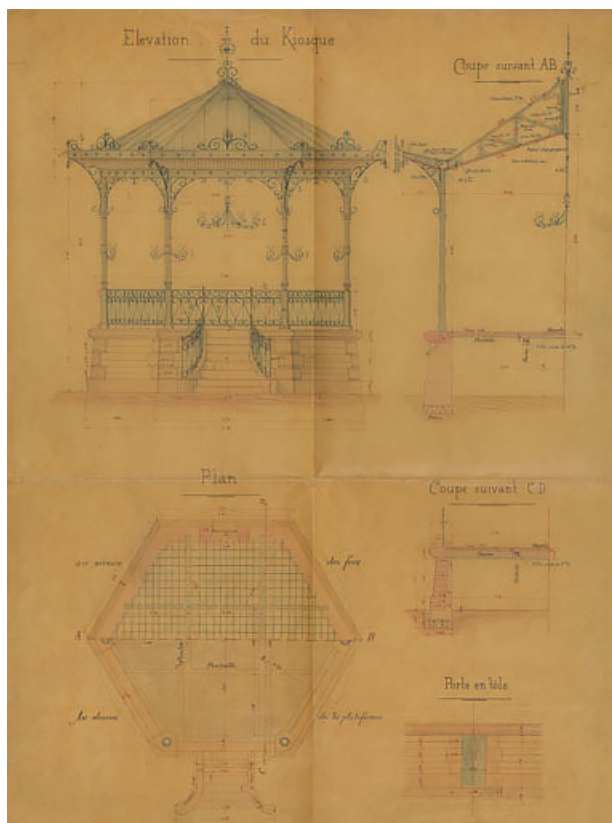
Ville de Châtillon-sur-Seine. Etablissement d'un kiosque à musique. Plan, Elévation et Coupes de l'ouvrage à exécuter. 9 novembre 1908.
