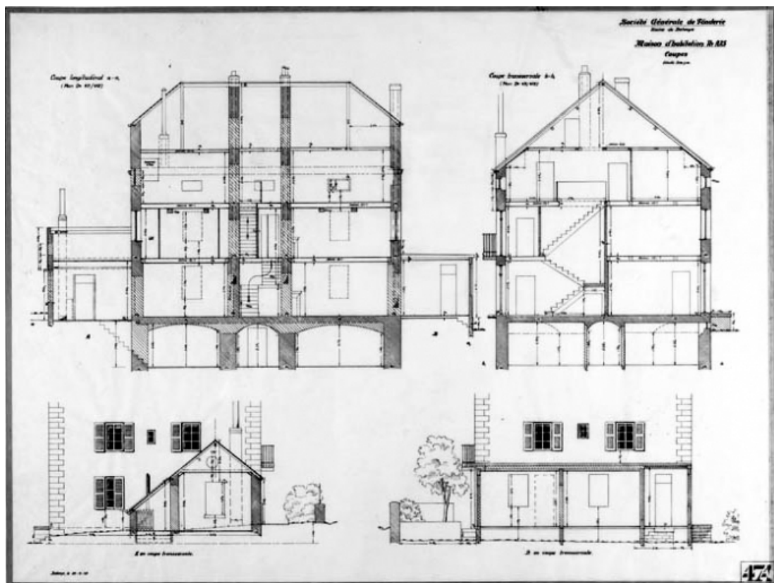
Société Générale de Fonderie. Usine de Belvoire. Maison d'habitation n° A25. Coupes.
