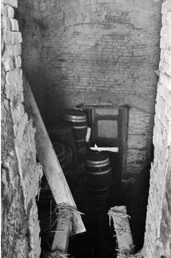
Intérieur du 1er four, depuis la porte d'enfournement. La voûte du foyer a été supprimée. 39, Vitreux
