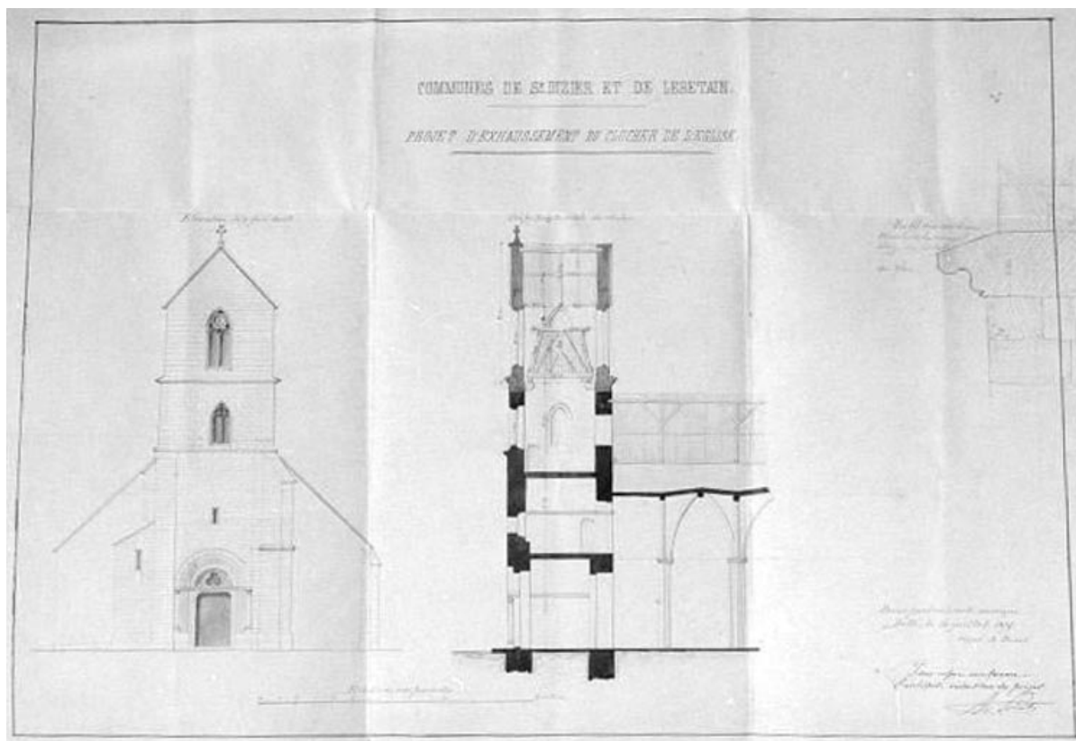
Projet d'exhaussement du clocher de l'église.
