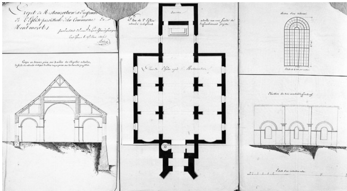
Projet de restauration et d'agrandissement de l'église paroissiale de la commune de Montmorot, vu avec la retombe du plan. 39, Montmorot montée de l' Eglise
