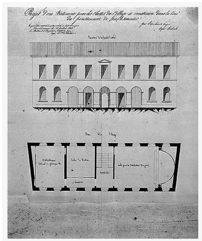
Plan et élévation du bâtiment annexe construit après 1828.
