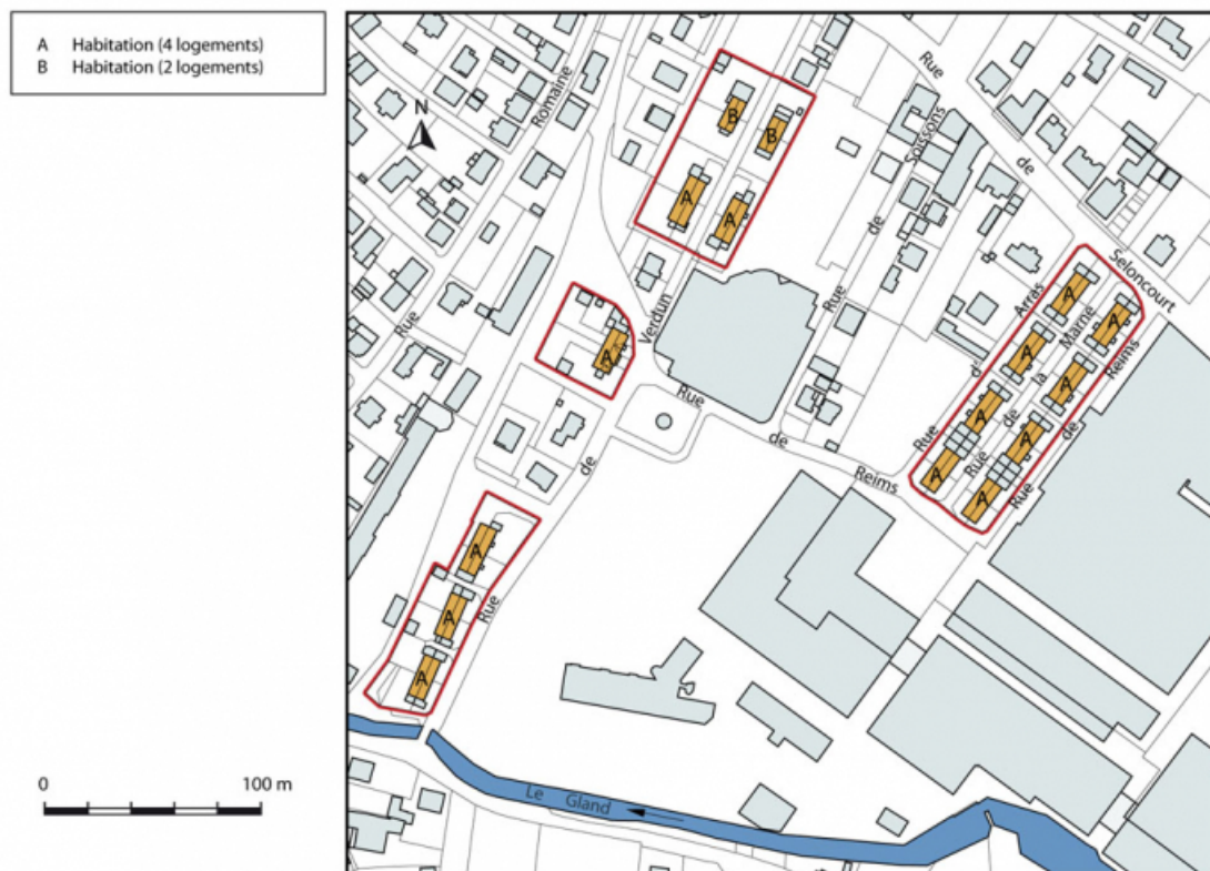
Plan-masse et de situation. 25, Audincourt rue de Verdun
