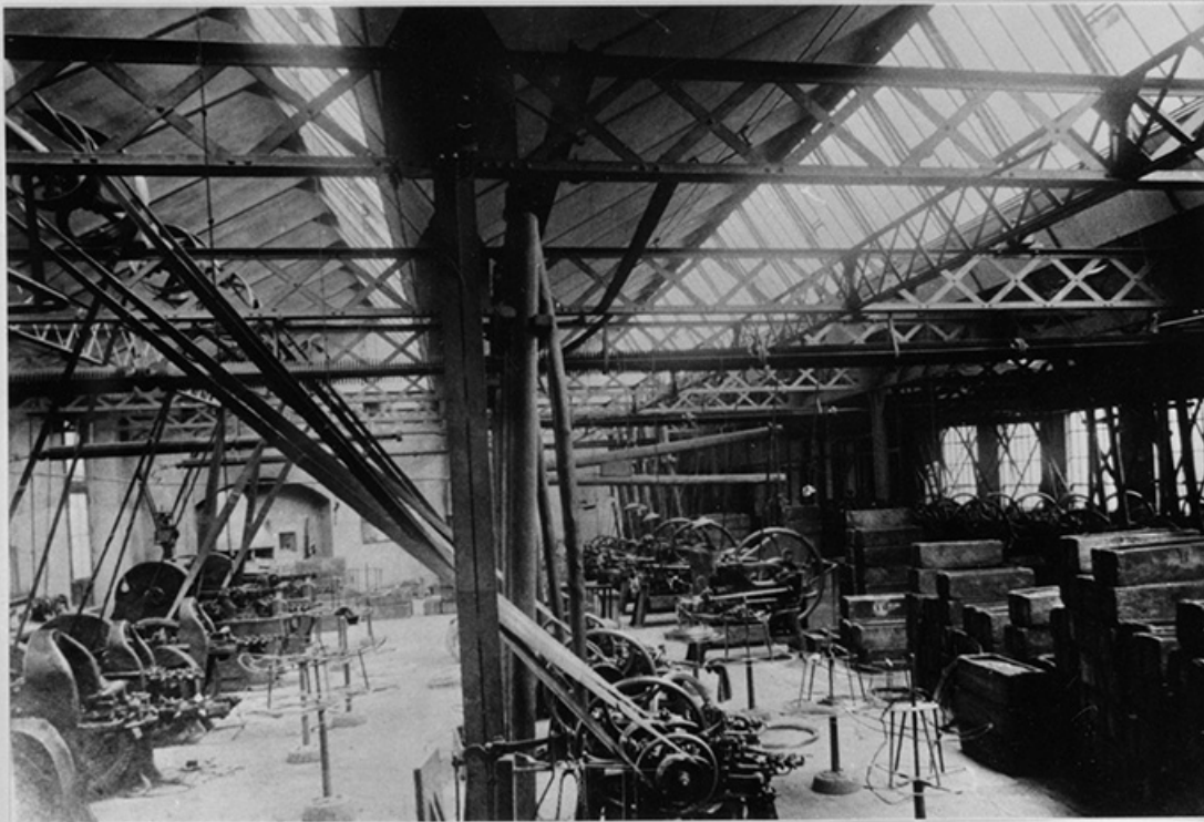
Intérieur de la clouterie : les tourets et les machines à clous, vers 1890-1900.
