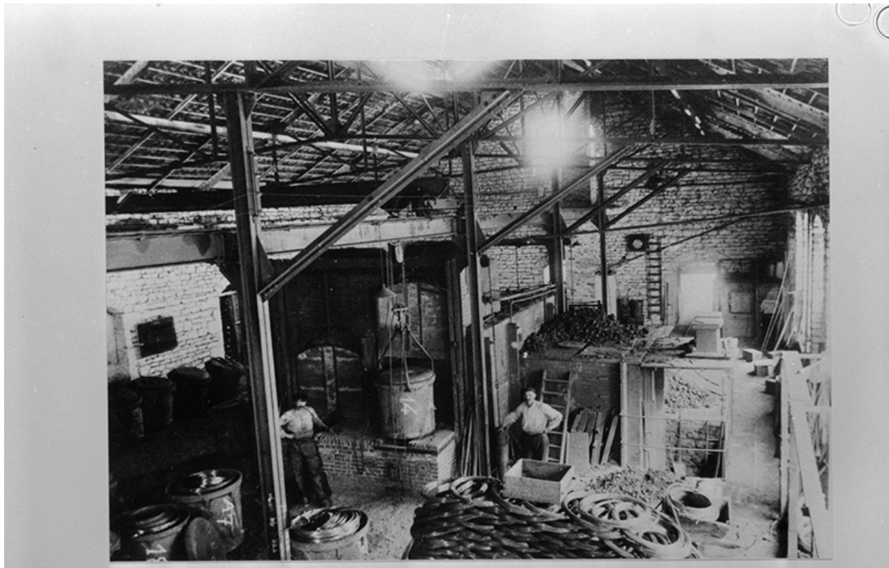
Intérieur du bâtiment abritant le "four à recuire" : l'entrée du four, vers 1890-1900.
