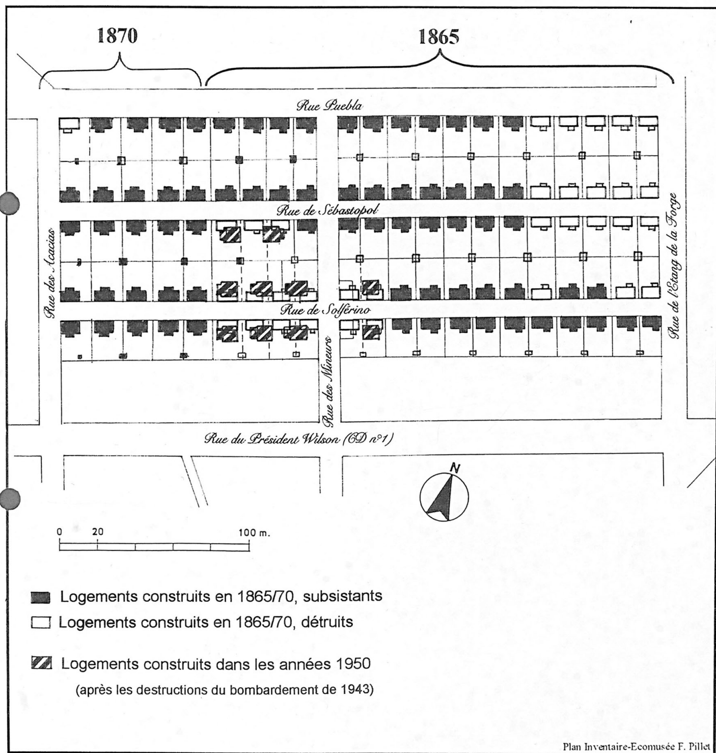
Pl. 3 : Plan-masse de la cité de la Villedieu en 2000 (ne tenant pas compte des remaniements et extensions des logements après construction), échelle 1/2000.
