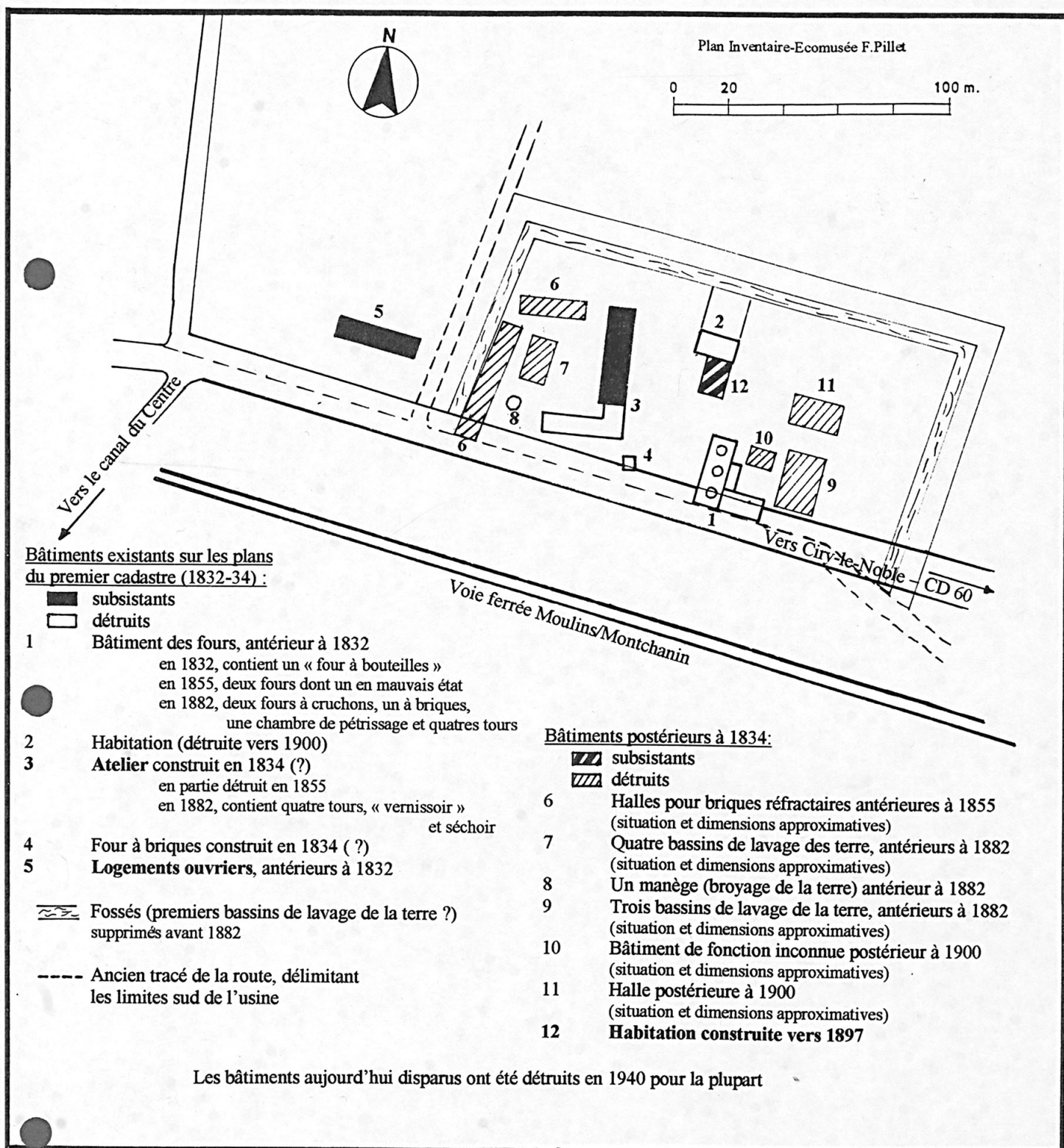
Pl. 3 : Plan-masse du site de l'usine de céramique de la Valteuse aux XIX e et XX e siècles, échelle 1/2000, plan Ecomusée-Inventaire F. Pillet.
