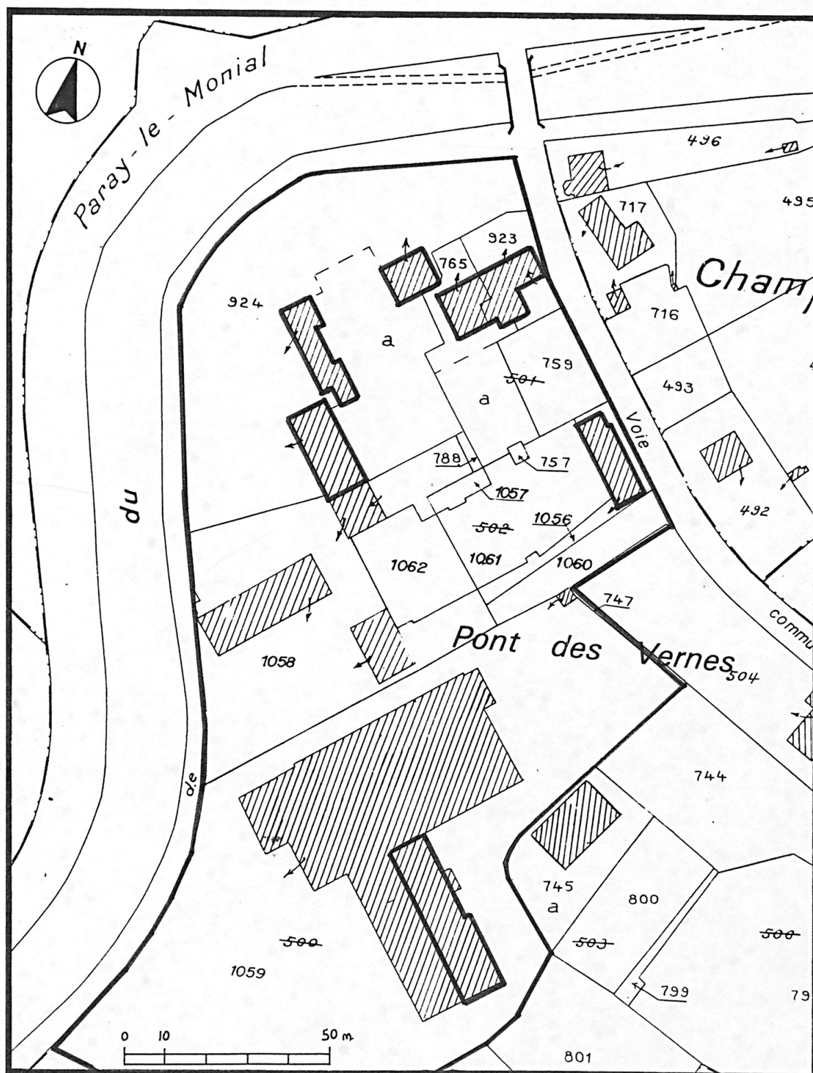
Pl. 2 : Plan de situation, extrait de plan cadastral, Pouilloux, section A3 , 1984, 1/1250.
