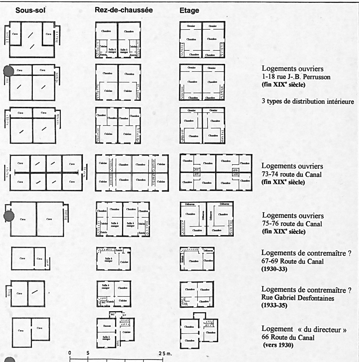
Pl. 4 : Plans des logements de la cité Perrusson construits de la fin du XIX e siècle à 1935, échelle 1/500, plan Inventaire-Ecomusée F.Pillet, d'après MICHAUD Claudine, Un site de l'industrie céramique en Saône-et-Loire : la tuilerie Perrusson et le hameau de la Neuvième-Écluse à Écuisses (1860-1960) , Mém. maîtr. Lyon II, Hist. de l'art. Dir. M me Perez, multigr., 1990, 204 p.
