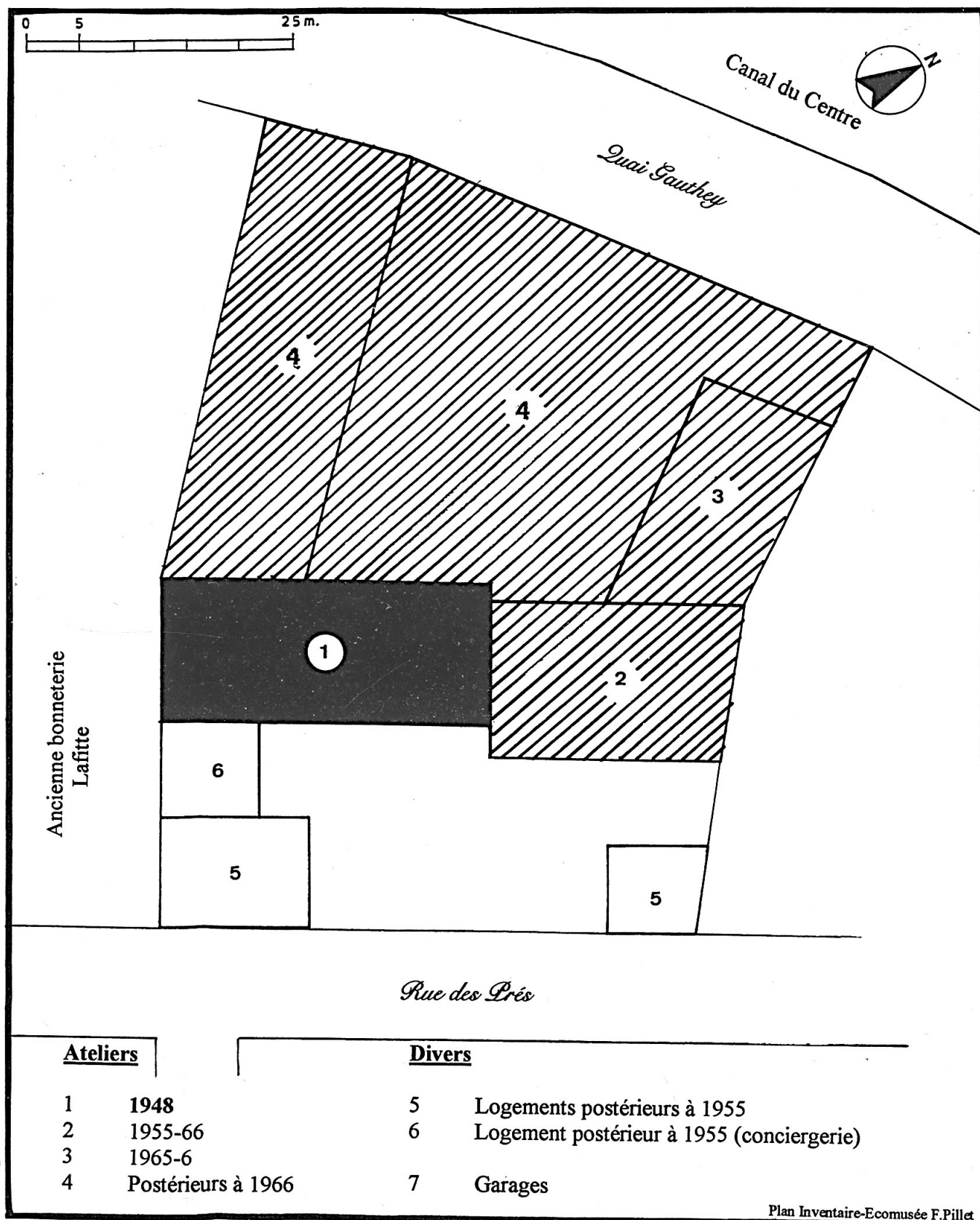
Pl. 3 : Plan-masse de l'usine de bonneterie Blanchard en 1999, échelle 1/500.
