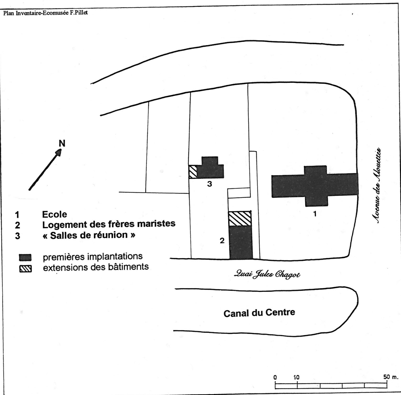
Pl. 3 : Plan-masse de l'ancienne école de la 9 ème écluse, échelle 1/1000.
