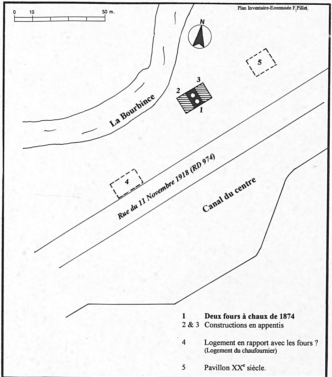
Pl. 3 : Plan-masse des fours à chaux, échelle 1/1000.
