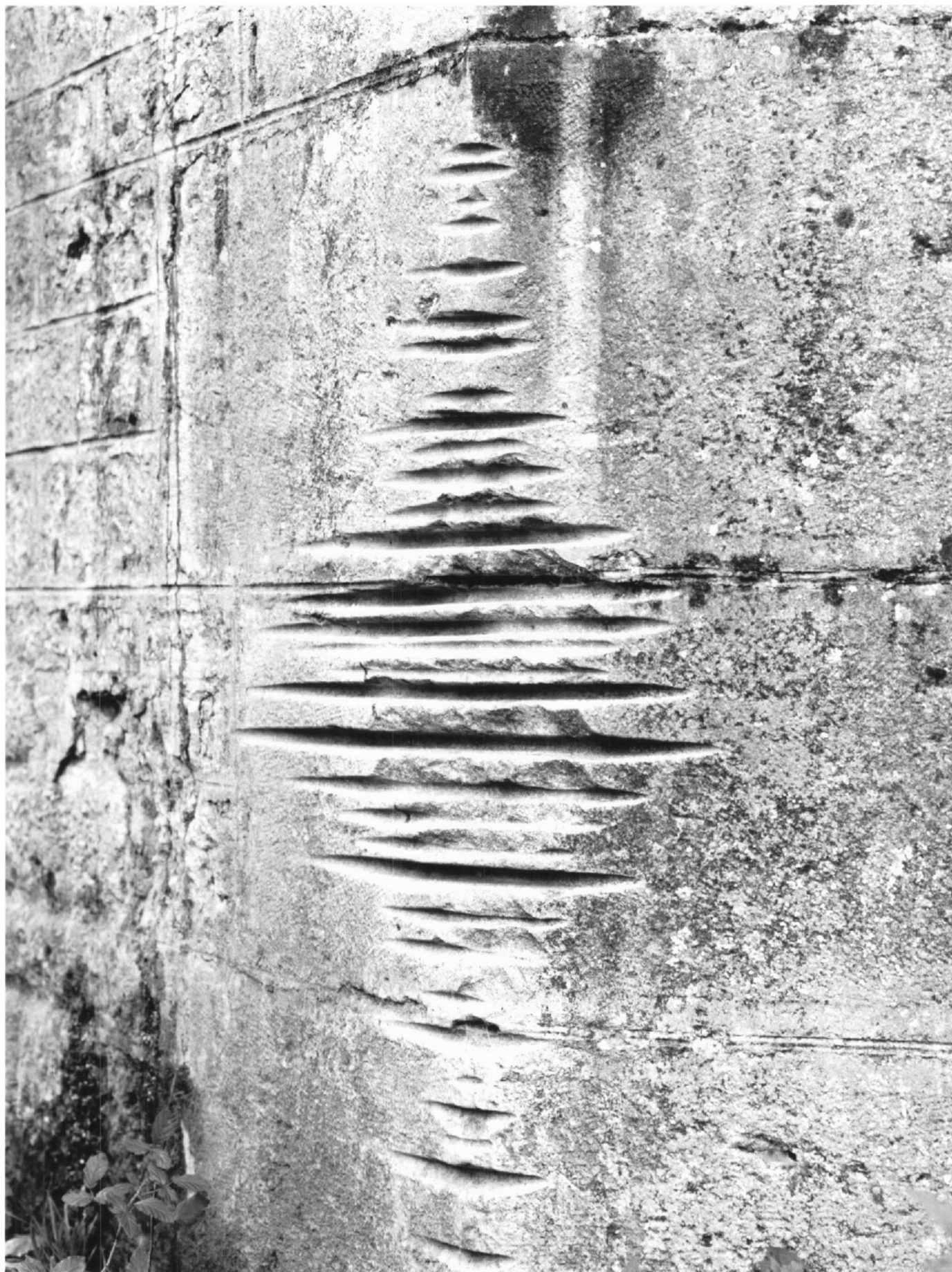
Fig. 002 Détail d'une arête de culée montrant les sillons dus aux frottements des câbles de halage
