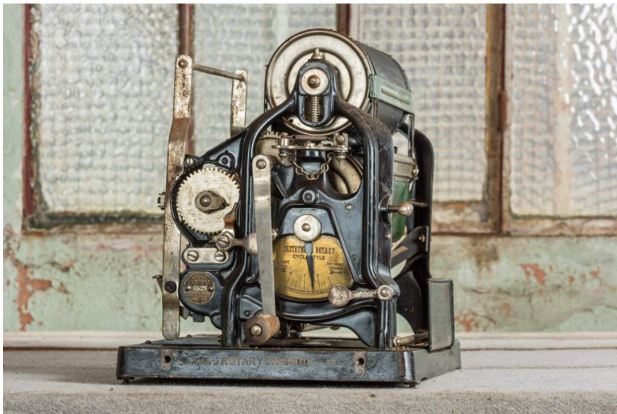
Face droite : poignée d'entraînement des cylindres et indicateur de pression. 71, La Clayette, 2A rue Faisant
