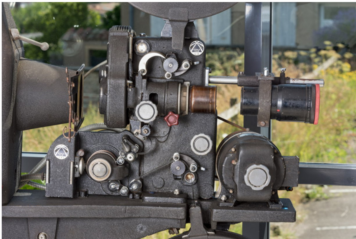
1er projecteur : chrono (bloc de projection, avec optique et moteur électrique). 71, La Clayette, 2A rue Faisant
