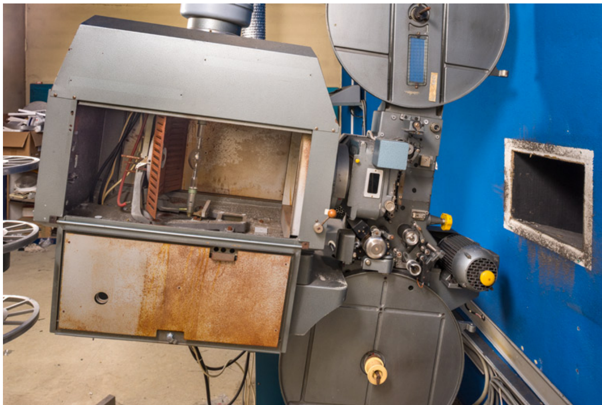
Projecteur : détail de la lanterne électrique ZX 2500 V et du chrono. 71, Montceau-les-Mines, 13 rue Ferrer
