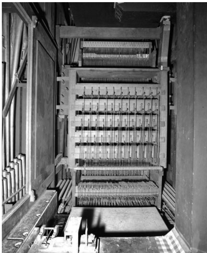
Mécanique de la machine pneumatique Barker.
