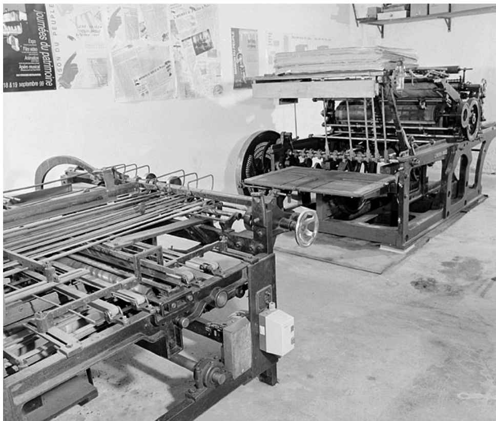
Vue d'ensemble de la pliuse Mentges et de la presse à cylindre Voirin.
