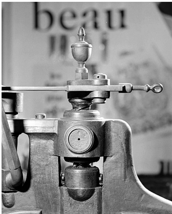
Partie supérieure de la vis, avec le système de transmission du mouvement du barreau.
