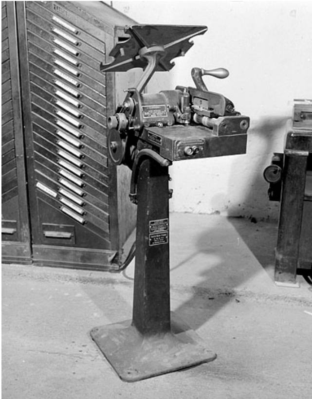
Vue d'ensemble d'une machine. Le support des lignes-blocs ("lutrins") est monté à l'envers (inclinaison vers l'arrière et non vers l'avant).
