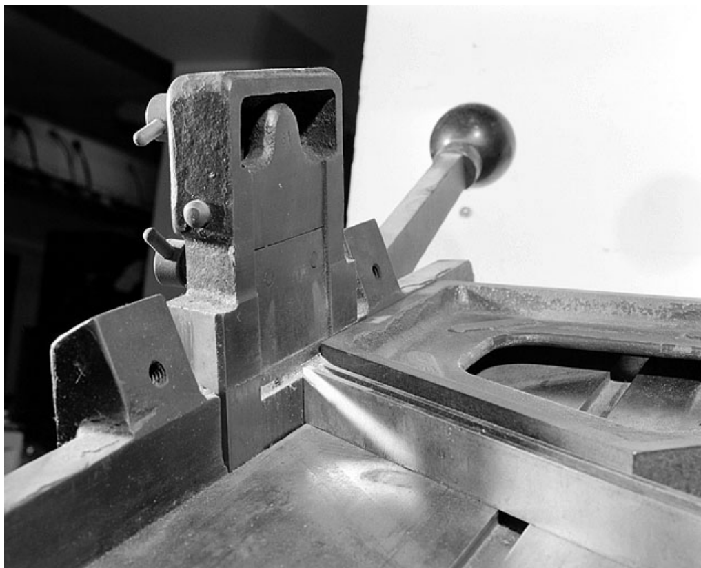
Coupe oblique d'un filet avec le "coupoir-biseautier". Le filet est appuyé contre le guide pentagonal. 39, Saint-Claude, 12 rue de la Poyat
