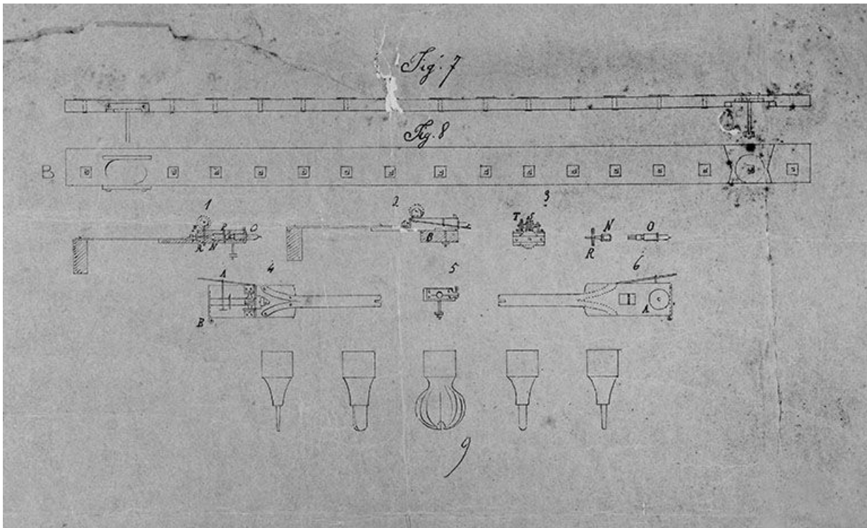
Dessins de détails : éléments du bâti, engrenages, système de rotation des supports d'ébauchons, fraises. 39, Saint-Claude, 19 rue Carnot
