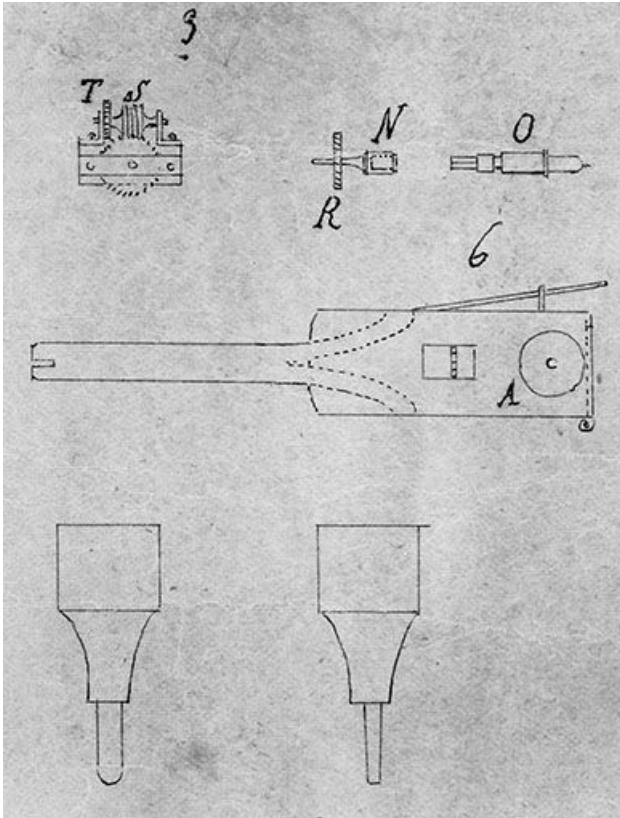
Dessins de détails [partie gauche du plan] : engrenages, système de rotation des supports d'ébauchons, fraises. 39, Saint-Claude, 19 rue Carnot
