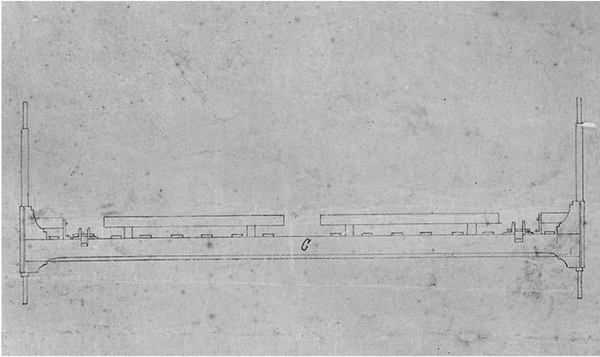
Élévation partielle de la face postérieure : détail du plan montrant une partie du bâti mobile.
