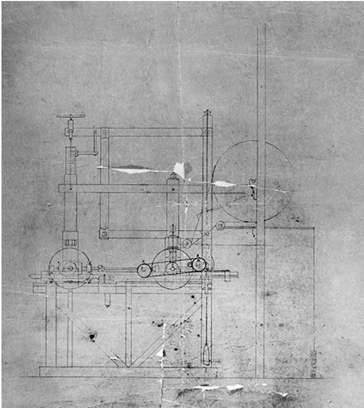
Élévation de la face latérale droite.
