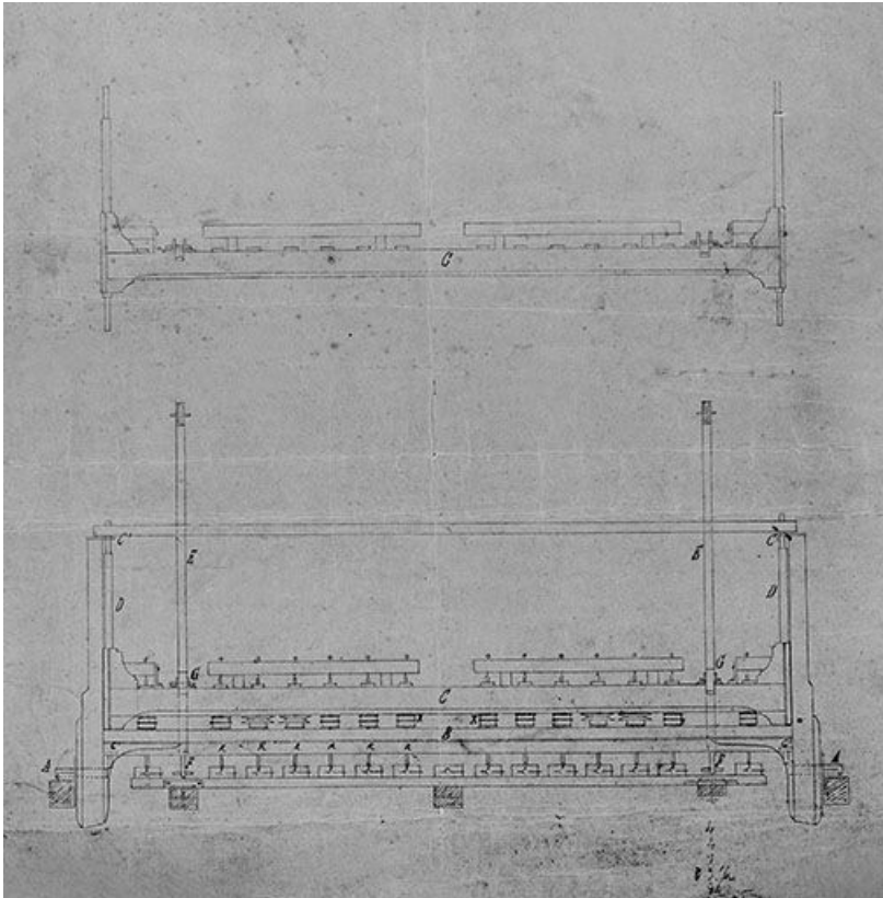
Élévation partielle de la face postérieure donnant les dessins du système d'entraînement des fraises et de fixation des ébauchons, et d'une partie du bâti mobile.
