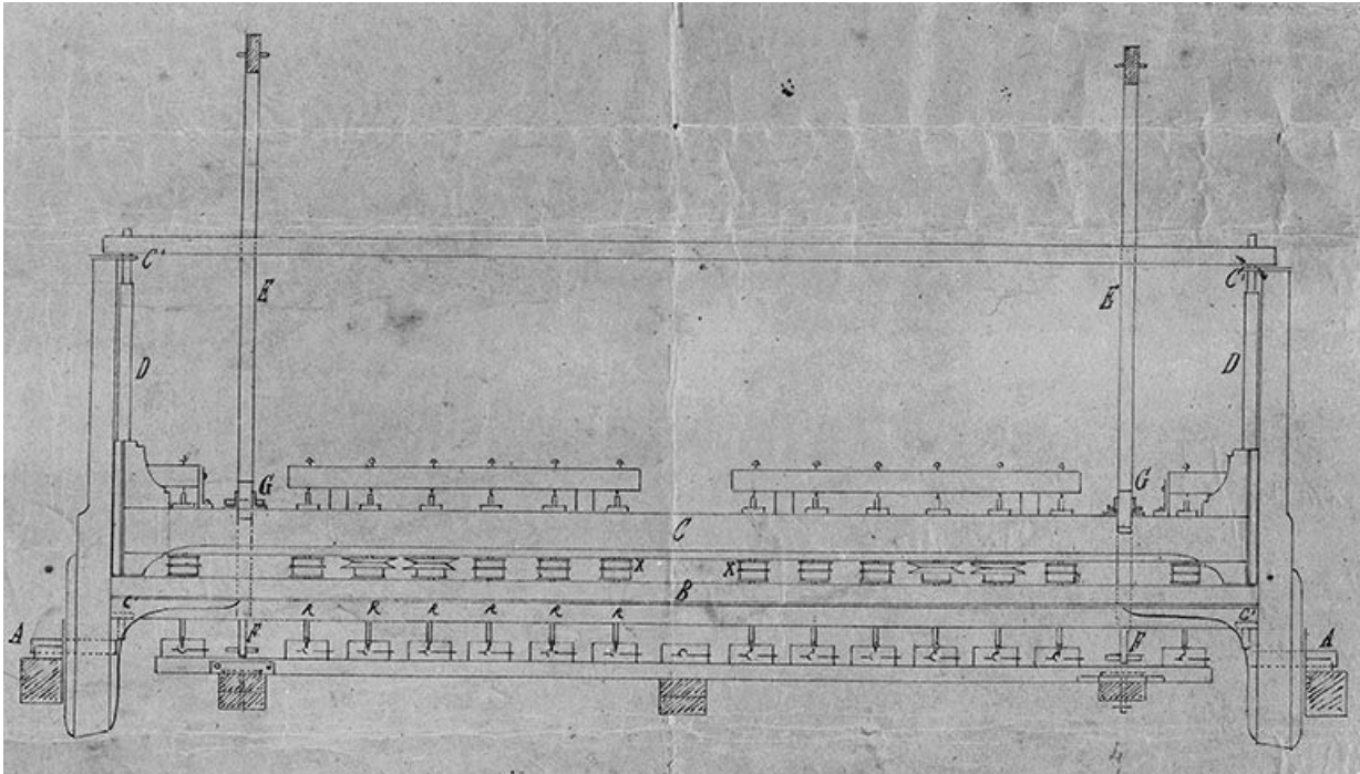
Élévation partielle de la face postérieure : détail du plan montrant le système d'entraînement des fraises et de fixation des ébauchons.
