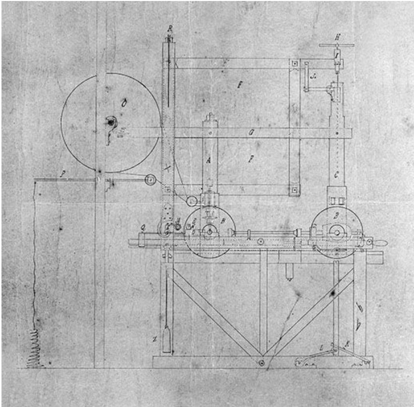
Élévation de la face latérale gauche.
