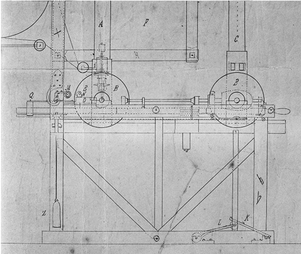
Élévation de la face latérale gauche : détail de la partie centrale du plan.
