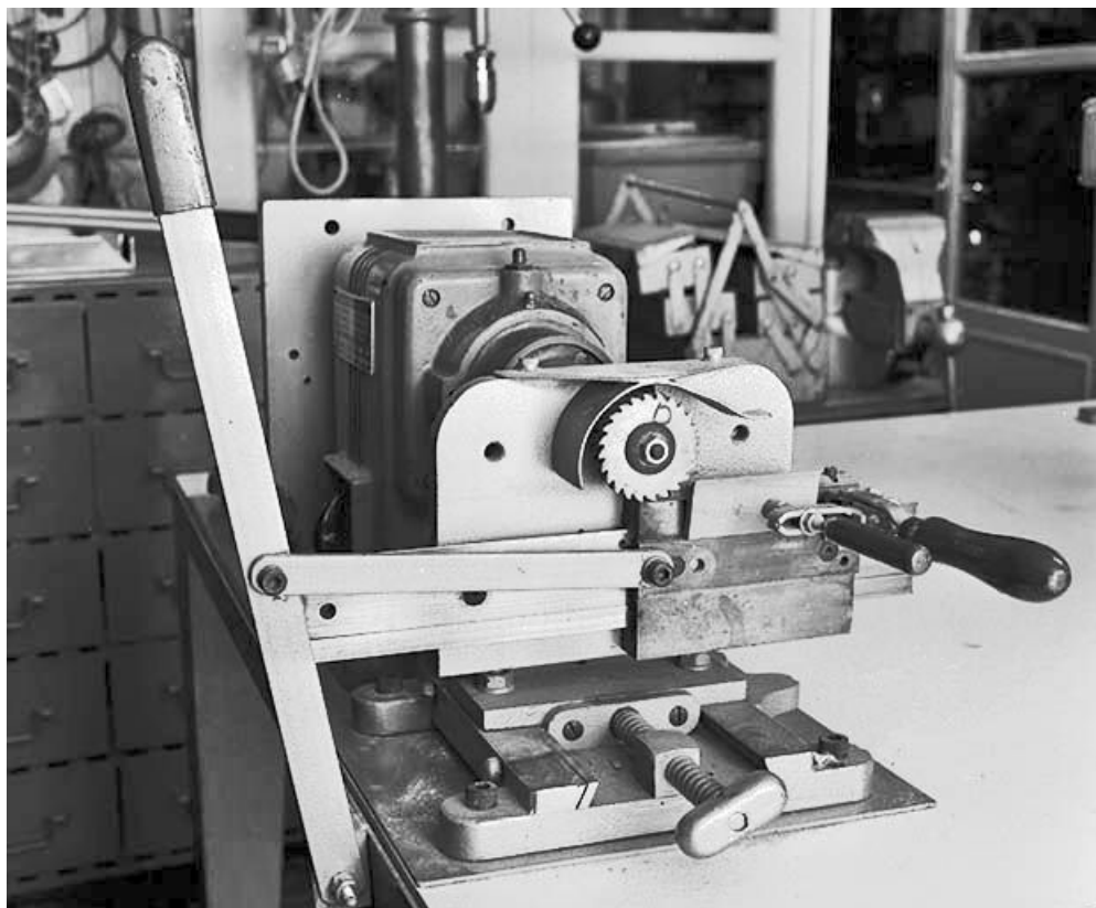
Détail de la fraise (côté fraiseuse).
