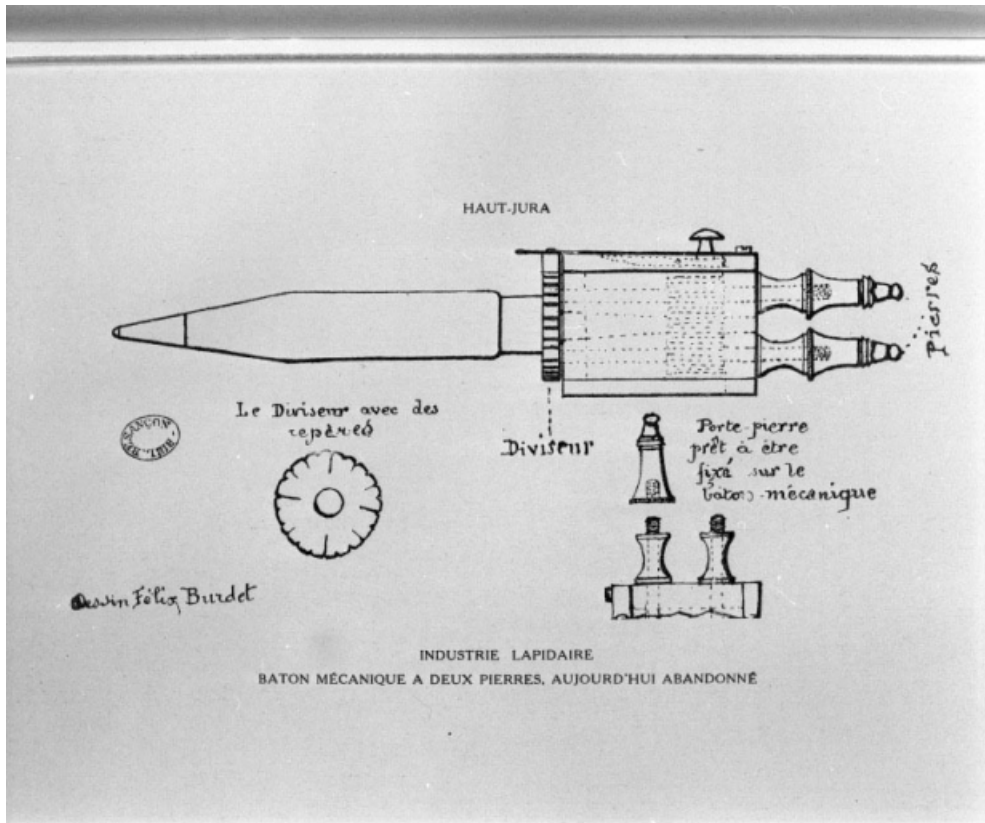
Bâton mécanique à deux pierres, aujourd'hui abandonné.
