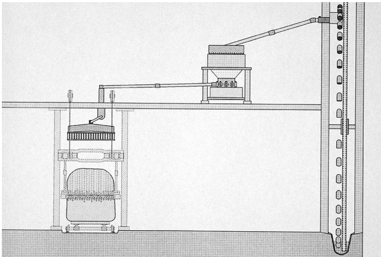
Schéma de fonctionnement de la norria et du système d'alimentation en " service " des châssis de scie.
