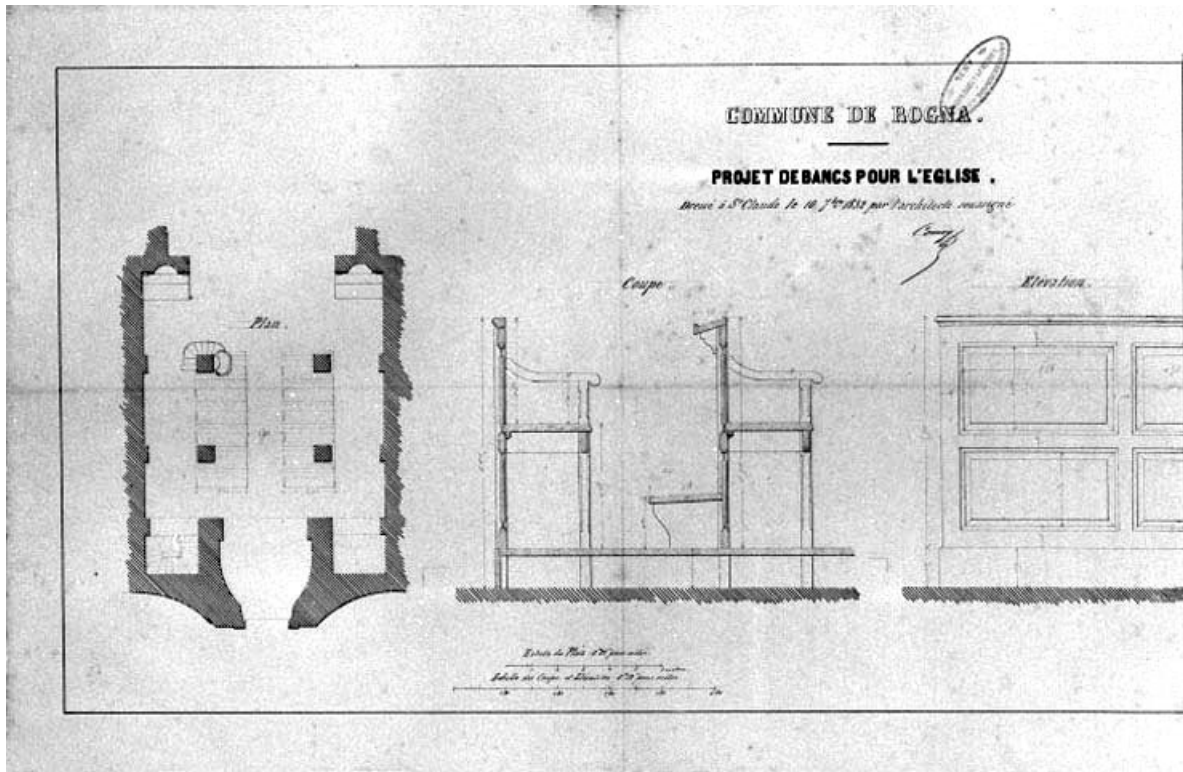
Commune de Rogna. Projet de bancs pour l'église [plan, coupe, élévation]. 39, Rogna
