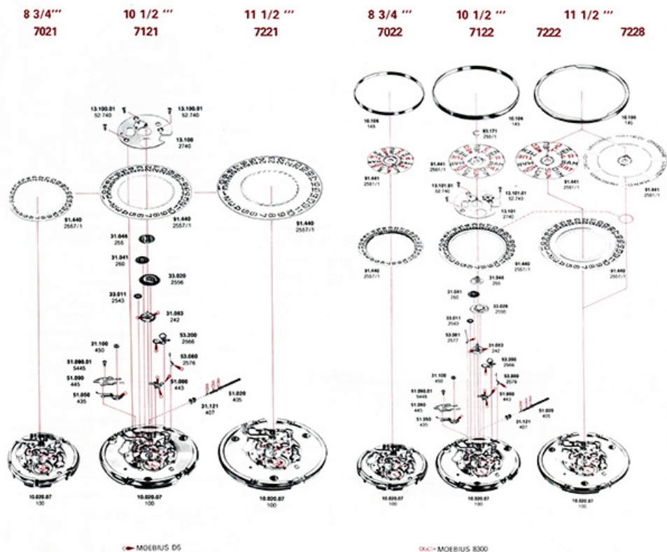
[Vue éclatée des mouvements FE 7020 7021 7022 7120 7121 7122 7220 7221 7222 7228 : affichage des jours et des quantième], 1988.
