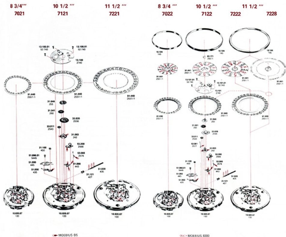
[Vue éclatée des mouvements FE 7020 7021 7022 7120 7121 7122 7220 7221 7222 7228 : affichage des jours et des quantièmes], 1988.
