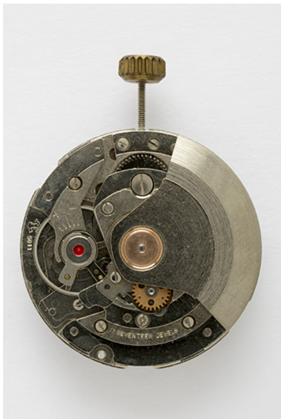
Mouvement France Ebauches FE 5611 : face côté ponts. 25, Villers-le-Lac
