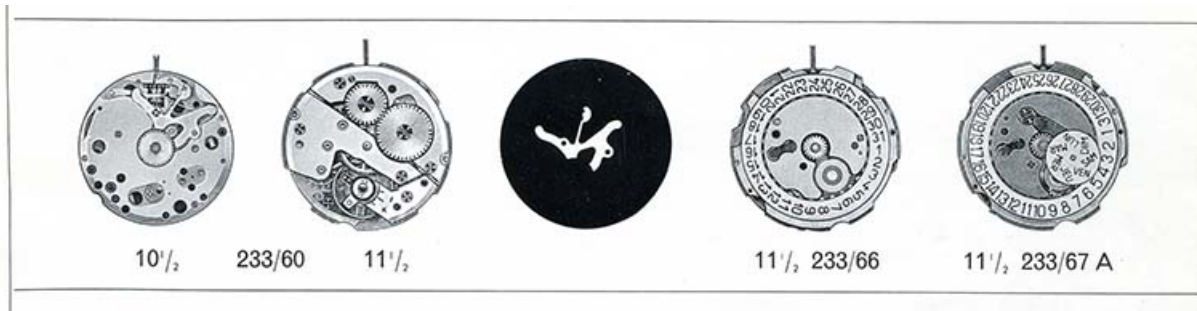
[Dessin des mouvements FE 233-60, 233-66 et 233-67A], 1973. 25, Maïche
