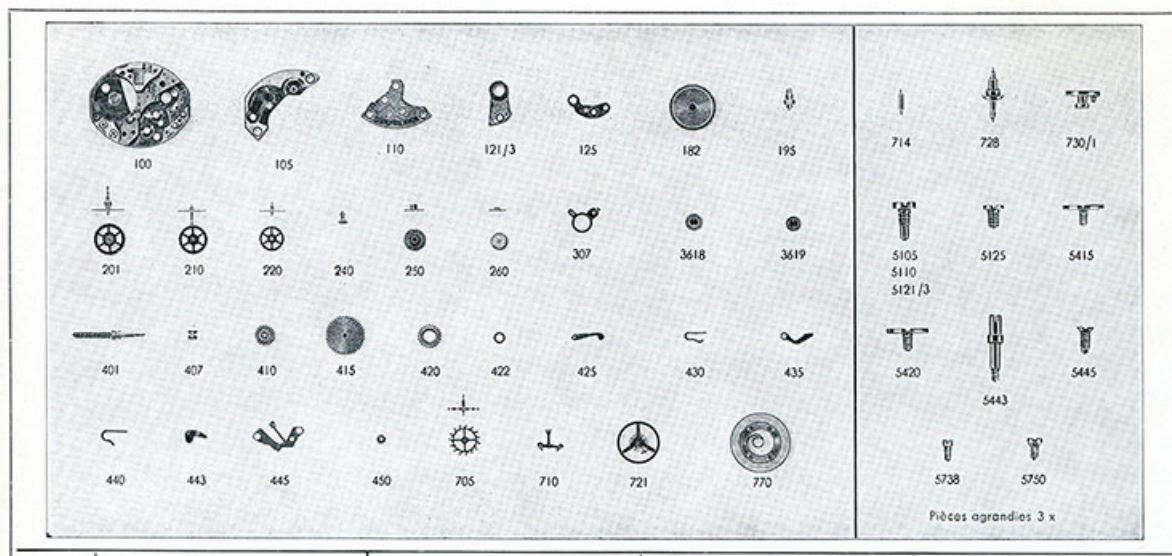
Calibre 5 1/2''' 68 - 17 rubis [éclaté des fournitures], 1973. 25, Maïche
