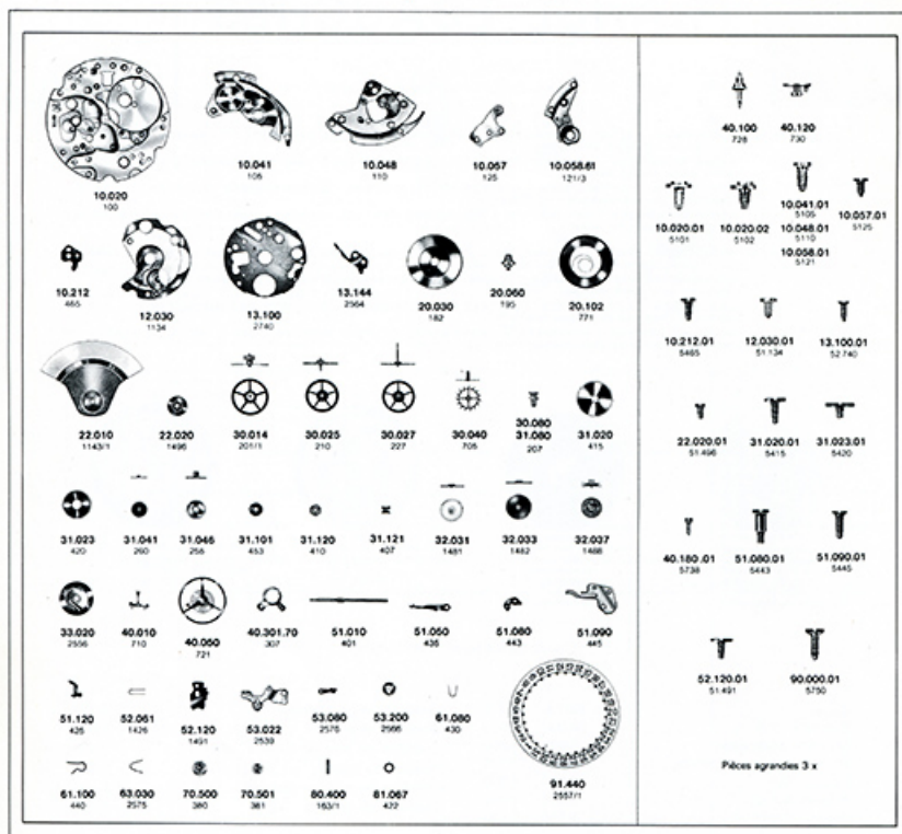
Calibre 11 1/2''' - 4611 A Automatique Calendrier [éclaté des fournitures], 1973. 25, Maïche
