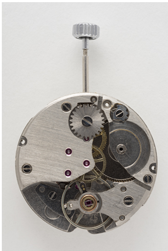
Mouvement FE 140-1, vu côté pont. 25, Maïche
