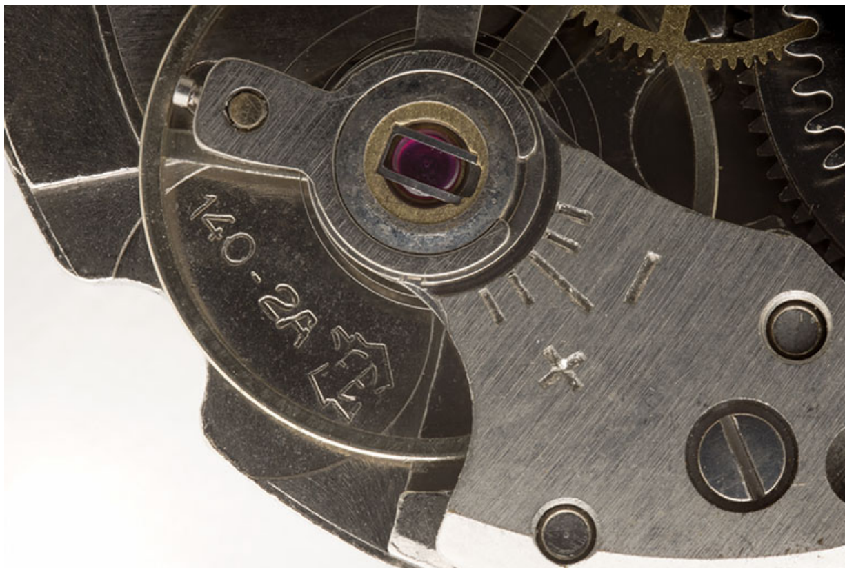
Mouvement de montre mécanique France Ebauches FE 140-2A : logotype de la société et indication du modèle. 25, Maïche
